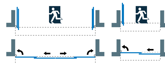
API doppi 2 ante scorrevoli 2 ante semi-fisse
