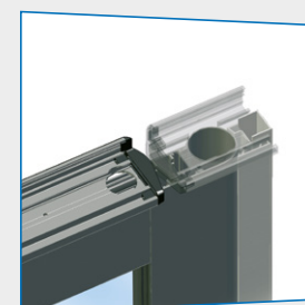
Profili anti-schiacciamento delle dita
