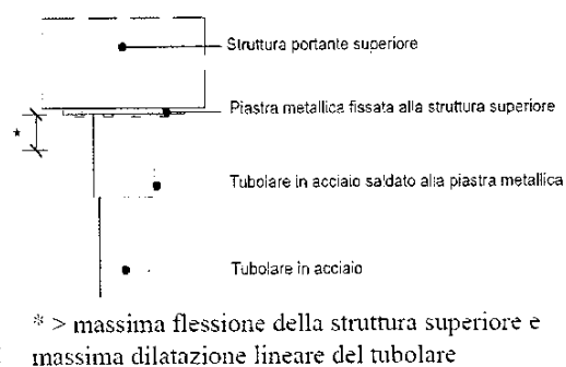
Figura 7: Irrigidimento con tubolare nello spessore del blocco, spessore medio (spessore tra 15 cm e 20 cm)
