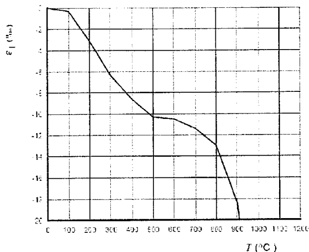
Figura 2: estratto da norma EN 12602-2016 - annex C - coefficiente \epsilon_T - andamento della deformazione termica del calcestruzzo cellulare in funzione della temperatura.
