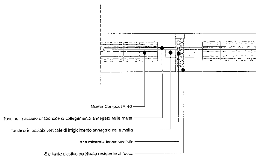
Figura 8: Irrigidimento con tendino inserito nello spessore del blocco nella posizione centrale per pareti in blocchi di piccolo spessore (blocchi spessore da 8 a 15 cm).
