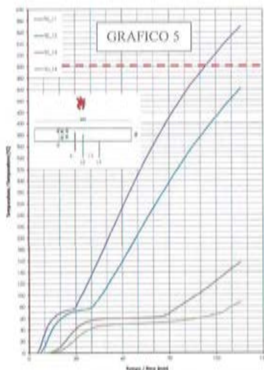
Grafico 5 - Andamento delle temperature delle termocoppie posizionate nello spessore nel blocco sp. 8 cm di densità 480 \text{ Kg/m}^3 (vedi schema posizionamento sopra riportato). - I dati sono stati estratti dal rapporto di prova CSI233MR. La curva viola è posizionata a 25 mm di profondità dalla faccia esposta al fuoco, quella blu a 40 mm di profondità e quella rossa a 65 mm di profondità dal lato esposto al fuoco.
